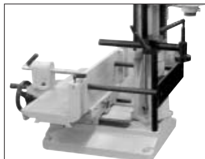
Cod articol 719 A-MDA - Set suport si presa pentru lucrari la inclinare de 180°
