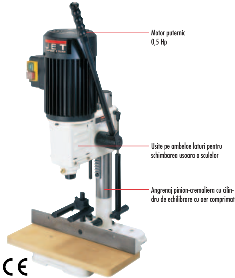
Frezare rapida si exacta pentru toate imbinarile de lemn si orice lacasuri pentru broaste si incuietori
